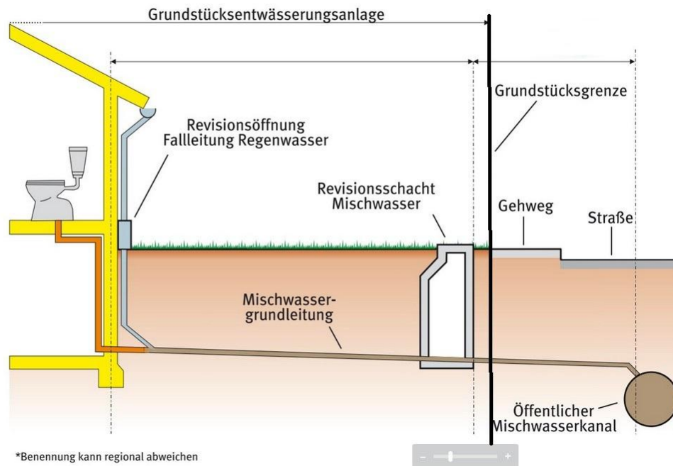
Systemskizze Mischsystem
